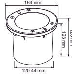
HLED-685/9W/30 CILLI
