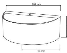
HLED-404/5W/40/S ANDORRA
