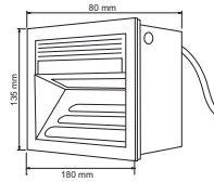
HLED-915/S TWER
