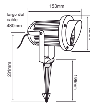
HLED-750/N BILBAU
