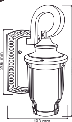
FTL-4000/BA ROMA
