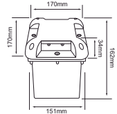
HLED-906/5W/30/S CALI
