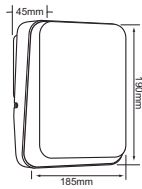
HLED-117/30/N ACANTHUS
