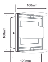
HLED-840 RAVENNE
