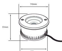
HLED-961/30 RUTA
