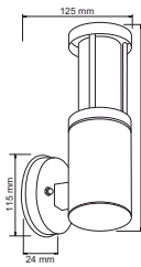
H-760/S TALLIN
