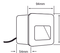
HLED-916/30/G CETI
