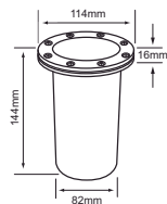
H-615/N CUENCA
