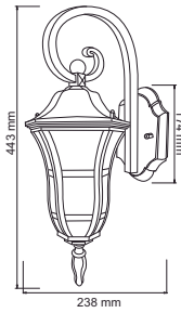
FTL-3300/BA SEGOVIA
