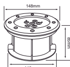
HLED-530/7.5W/30 CHICAGO
