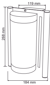
H-1050/S VENEZIA
