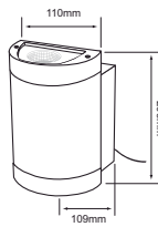
HLED-844/30/CR EDULIS
