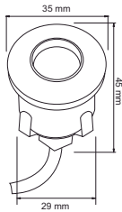
HLED-635/S CASTI
