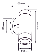
HLED-761/S ZINNER
