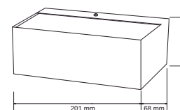
HLED-404/5W/40/S ANDORRA
