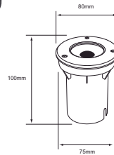
HLED-650/12W/30 CALICUT
