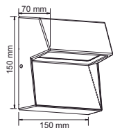
HLED-405/5W/40/S ABUYA
