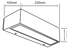
HLED-410/20W/40 AACHEN
