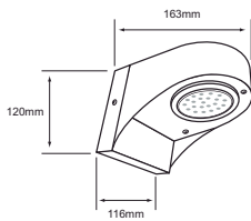
HLED-190/AN CINTU
