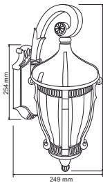
FTL-4100/BA TERME
