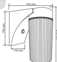
GL-20 VICENZA
