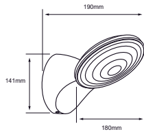
HLED-1152/G PERSEIDA
