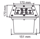
HLED-645/2W/S BARATI
