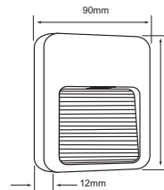
HLED-941/30/B ESFERIS
