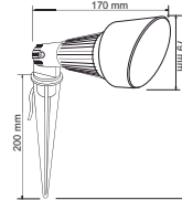
H-750/V BILBAO
