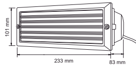
H-930/B CASTILLO
