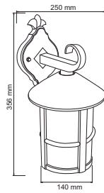
FTL-3420/S POZNA
