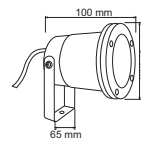
H-510/S ESCALONA
